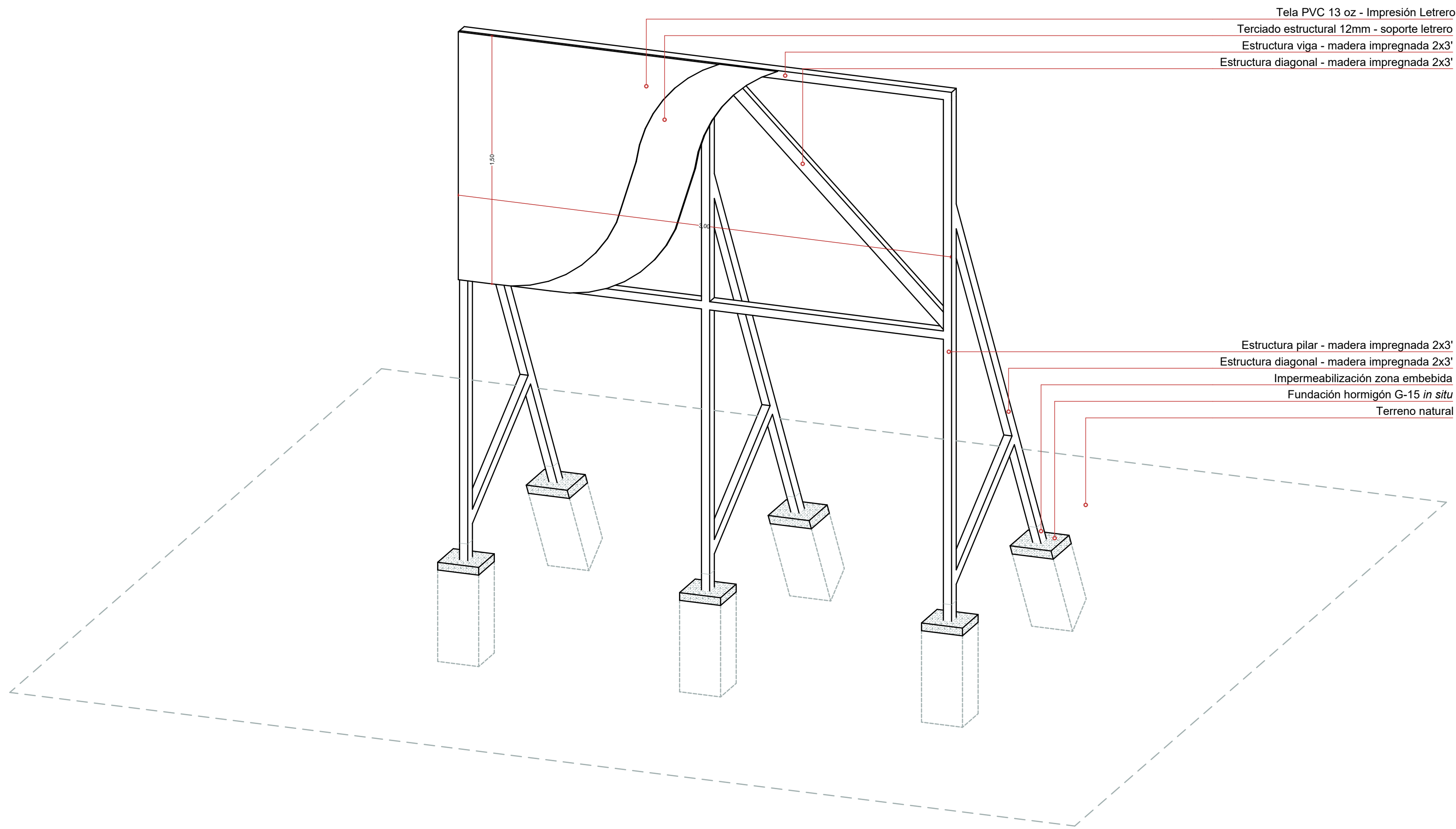
Diagrama axonométrica
